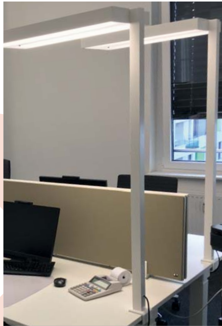
Bürobeleuchtung eines Büros in Freiburg mit Stehleuchten, an höhenverstellbaren Tischen montiert
